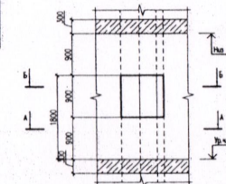
РАЗВЕРТКА УЧАСТКА СТЕНЫ С ЭЛЕКТРОЩИТОМ (проем 9)
