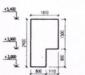
СХЕМА ПРОЕМА МАРКИ "4"
