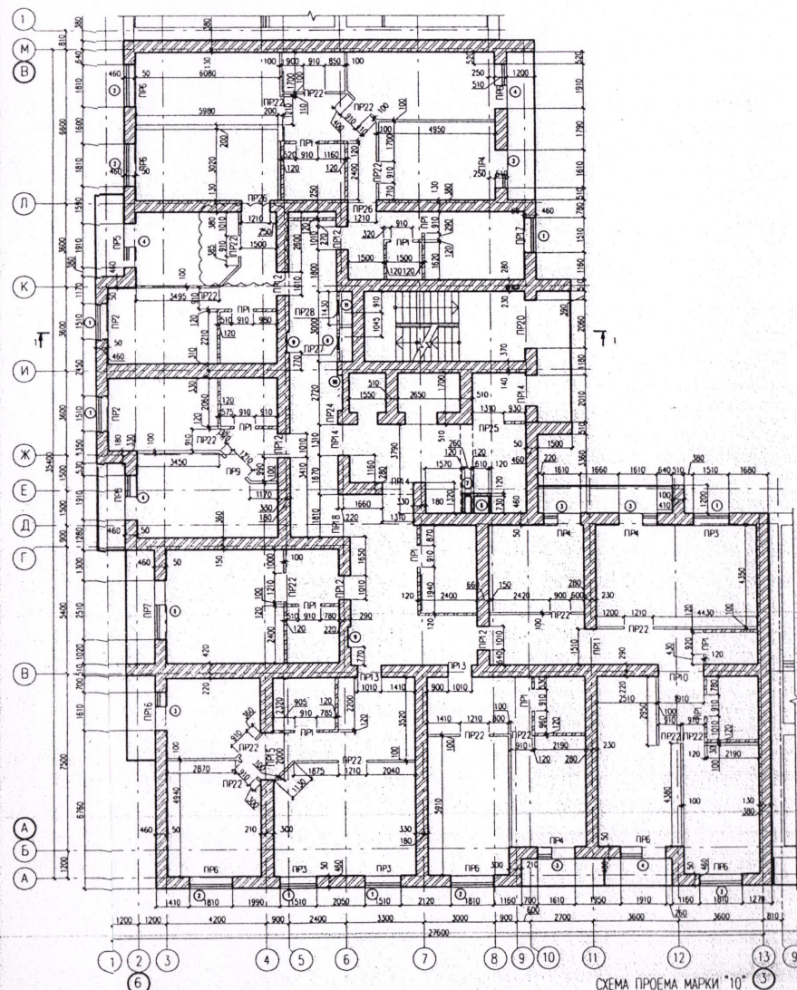
СХЕМА ПРОЕМА МАРКИ "10" (3)
