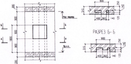
РАЗВЕРТКА ЧАСТИ СТЕНЫ С ЭЛЕКТРОЩИТОМ (проем 9)
