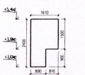
СХЕМА ПРОЕМА МАРКИ "3"
