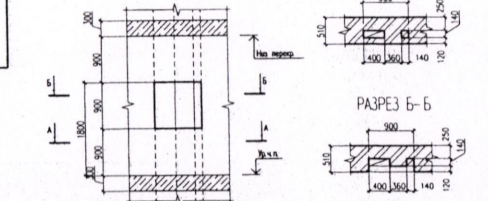
РАЗВЕРКА УЧАСТКА СТЕНЫ С ЭЛЕКТРОПРОТОМ (проем 9)
